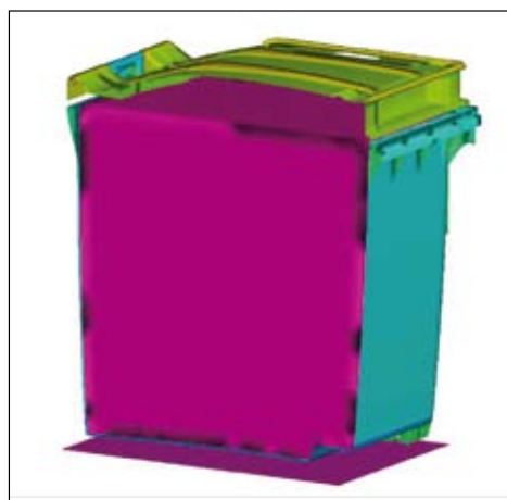
Finite Elemente Stoßsimulation: Simulation des Falltests für einen Müllgroßbehälter
